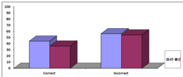
Fig 3: Affricates
